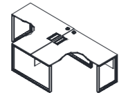
两人 L 工作位主桌 DL62-2.GJ W1400*D2812*H750 W1500*D3012*H750 W1600*D3212*H750
