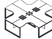
四人 L 工作位主桌 DL63-2.GJ W2812*D2812*H750 W3012*D3012*H750 W3212*D3212*H750
