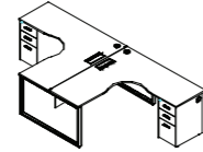
两人 L 工作位主桌 DL62-2.CG W1400*D2812*H750 W1500*D3012*H750 W1600*D3212*H750
