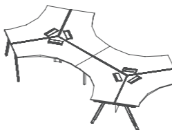
DN51 W4716•D2710•H750(mm)
